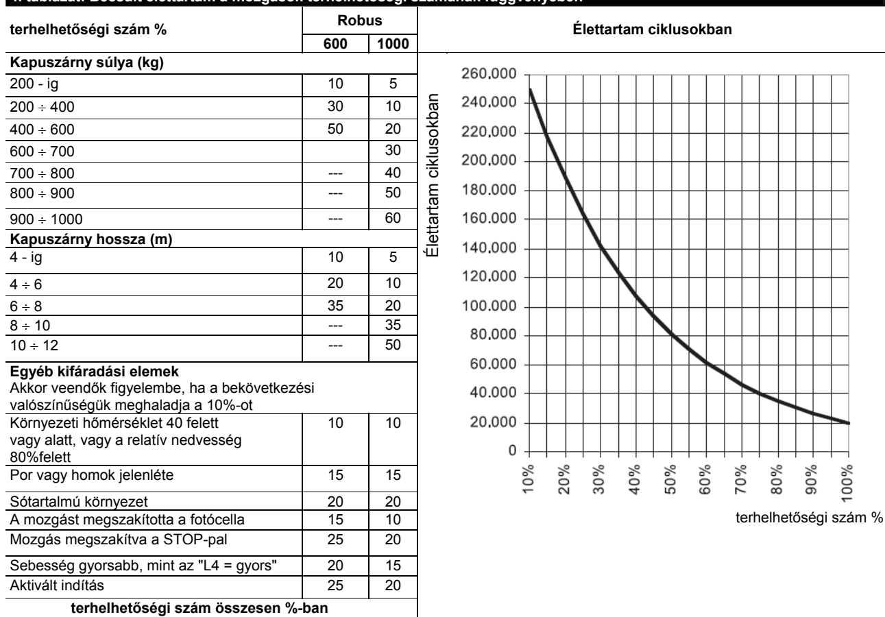
4. táblázat: Becsült élettartam a mozgások terhelhetőségi számának függvényében
